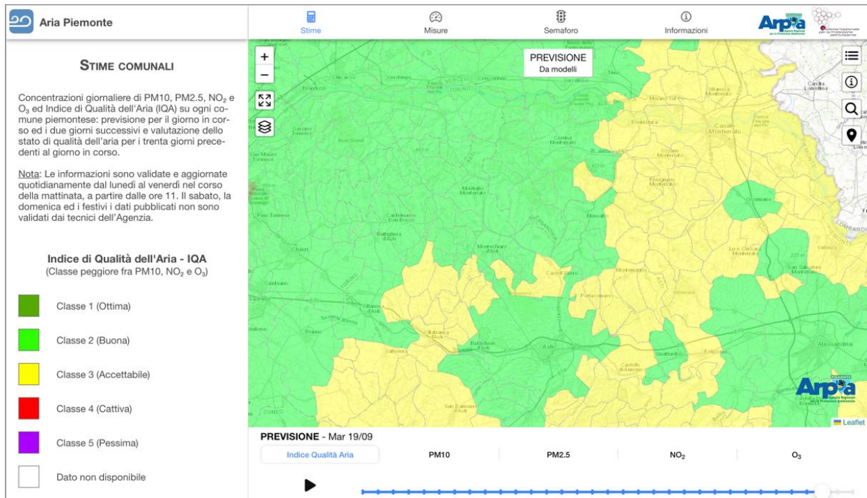
Grafico 26: Indice di Qualità dell’Aria (fonte: Relazione sullo stato dell’Ambiente – Arpa Piemonte 2023)
