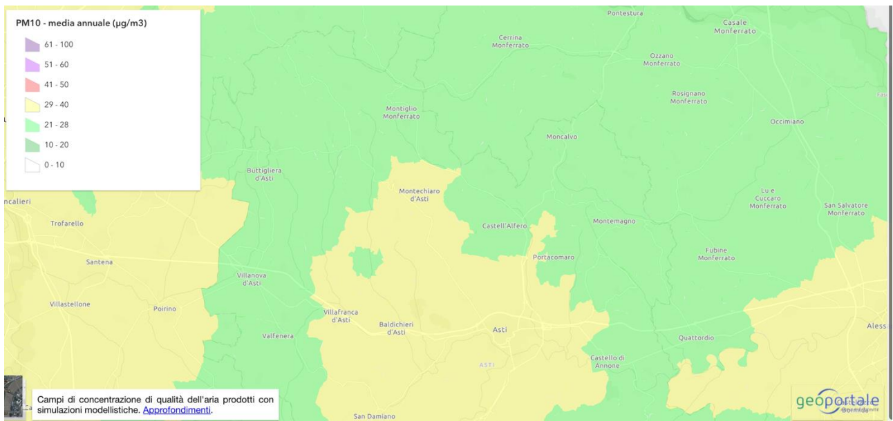
Grafico 29: PM10, media annuale 2022 (fonte: Relazione sullo stato dell'Ambiente – Arpa Piemonte 2023)
