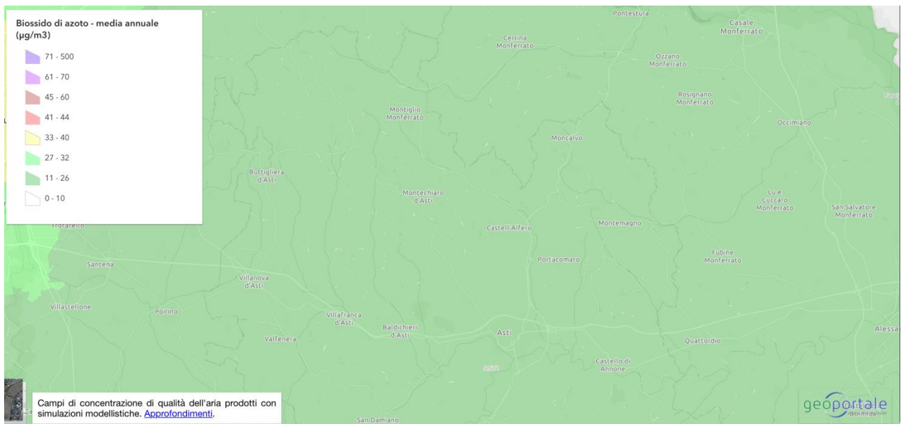
Grafico 27: Biossido di azoto, media annuale 2022 (fonte: Relazione sullo stato dell’Ambiente – Arpa Piemonte 2023)
